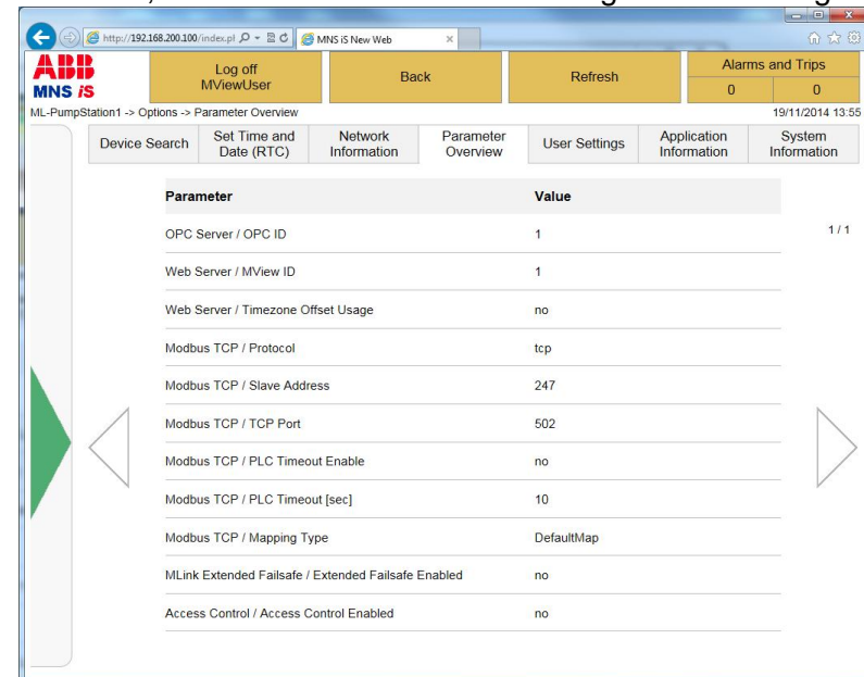
Figure 90 Parameter Overview - MLink
